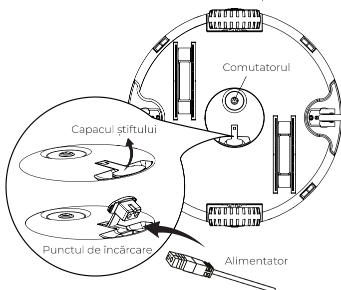
Ansamblul capacului de fund
