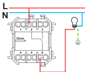
MONTAGE INTERRUPTEUR SIMPLE
