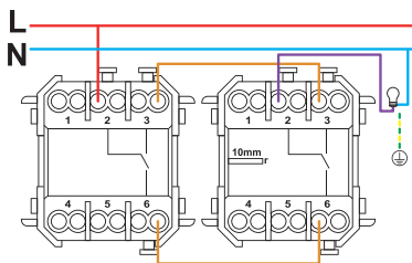
MONTAGE TYPE VA ET VIENT
