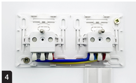
4 Fixer le support sur le mur
