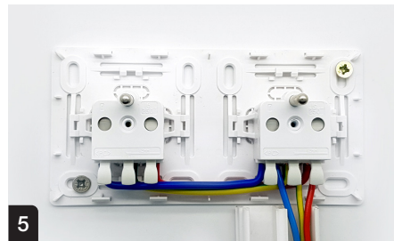
5 Effectuer le câblage directement sur le support
