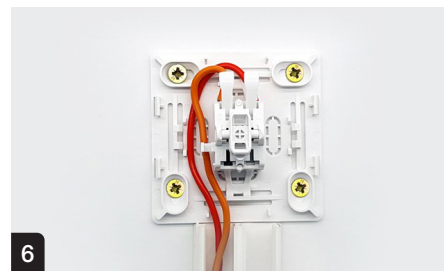
6 Effectuer le câblage puis clipser le mécanisme sur le support
