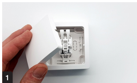
1 Déclipser la touche
