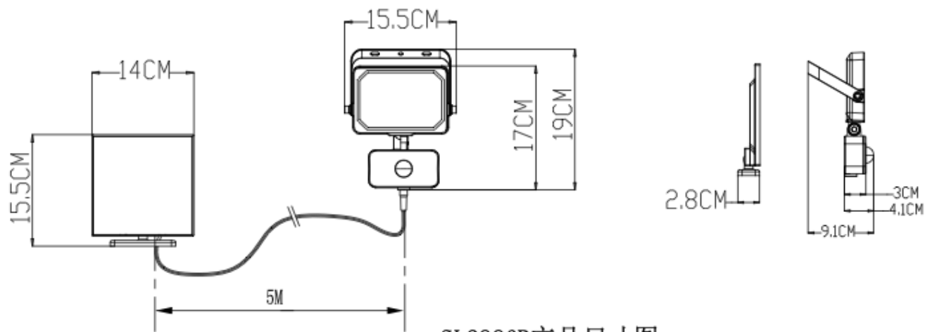
SL2886B产品尺寸图
