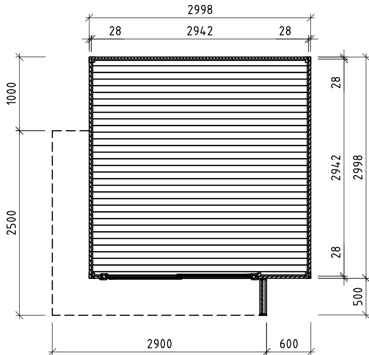
Grundriss
